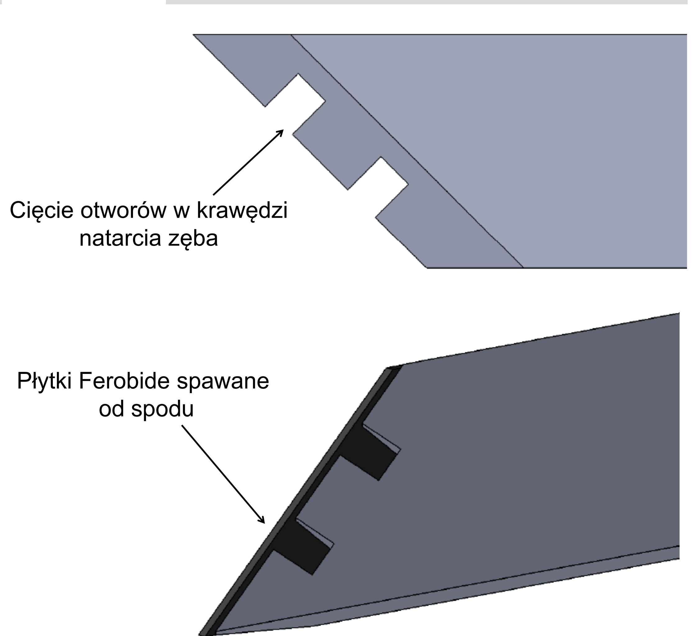
Otwory w części pługa
