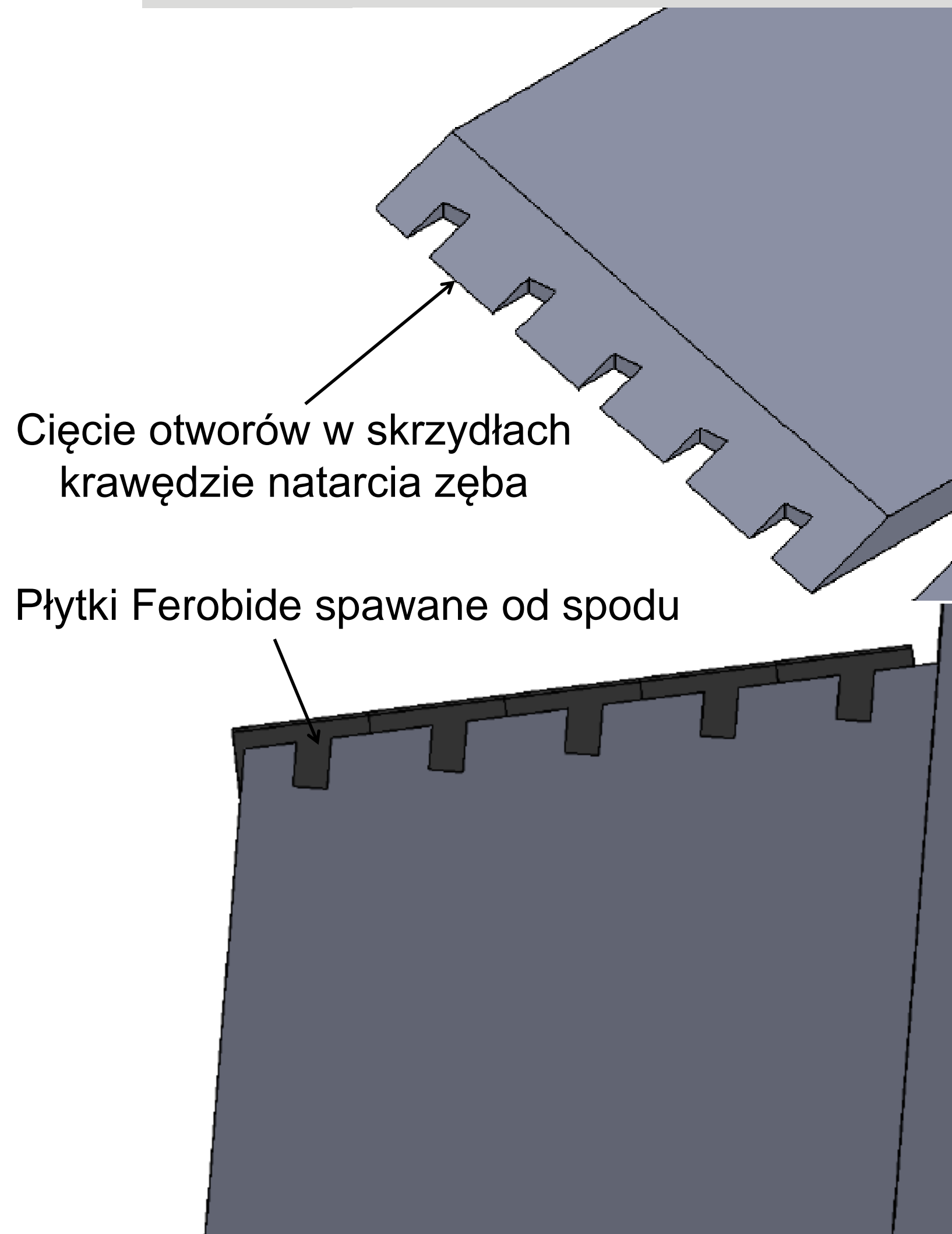
Otwory w zębach głębosza
