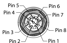
M12-A 8 pin
