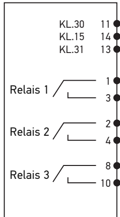
Blockschaltbild
