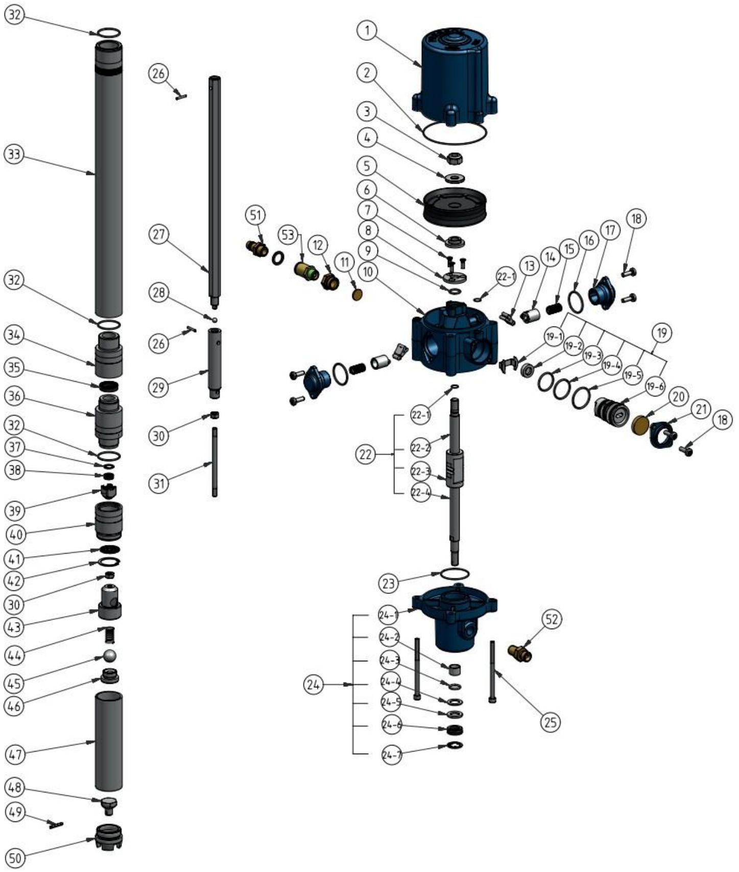
Afb. 13-1: Explosieaanzicht
