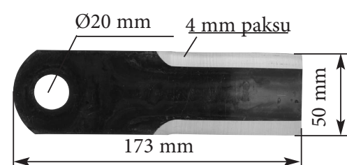
3025-736872 Pyörivä terä Sopii Claas - malleille
