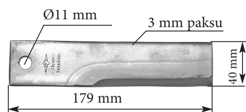
3605-0475 Vastaterä Sopii Rekordille
