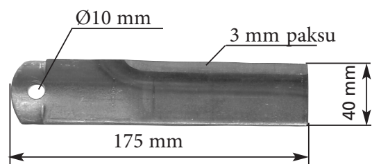
3605-0472 Vastaterä Sopii Rekordille
