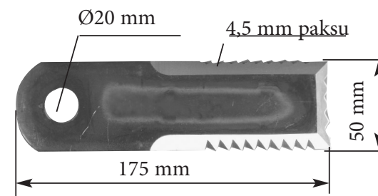
3605-0555-ORT Pyörivä terä, rihlattu sopii Rekordille
