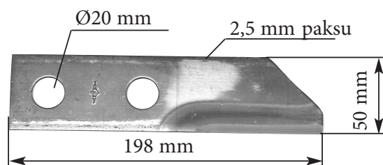
3605-0474 Pyörivä terä Sopii Rekordille
