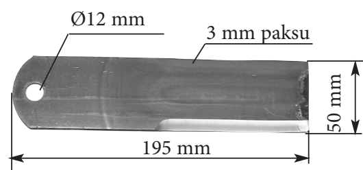
3605-0565 Vastaterä Sopii Claas ja John Deere -malleille
