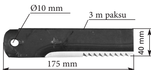
3605-0476-OR Vastaterä, rihlattu Sopii Rekordille
