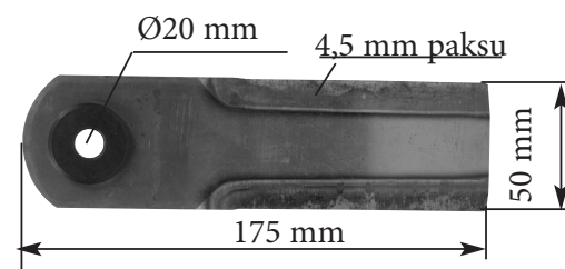
3605-0501 Pyörivä terä jossa pusla Sopii Case IH - malleille
