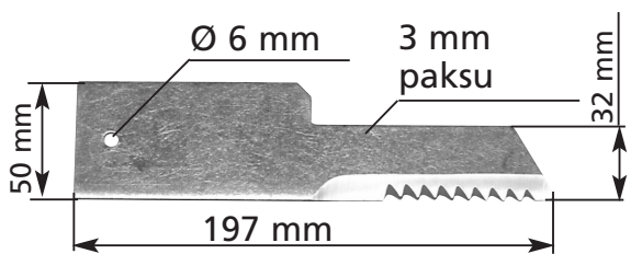
3605-0567-OR Vastaterä, hammastettu
