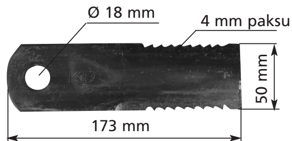
3605-0666-OR Pyörivä ja hammastettu terä Sopii KPAB:n silppurille
