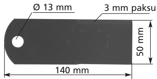
3605-0672 Vastaterä Sopii KPAB:n silppurille
