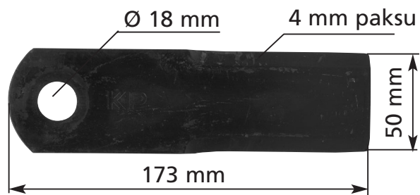
3605-0666 Pyörivä terä Sopii KPAB:n silppurille
