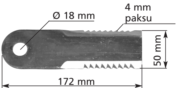
3605-0566-OR Pyörivä ja hammastettu terä
