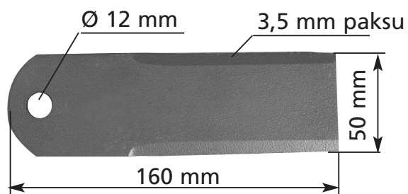
3605-0667 Vastaterä Sopii KPAB:n silppurille
