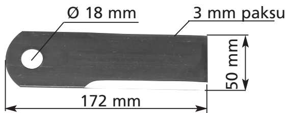
3605-0566 Pyörivä terä
