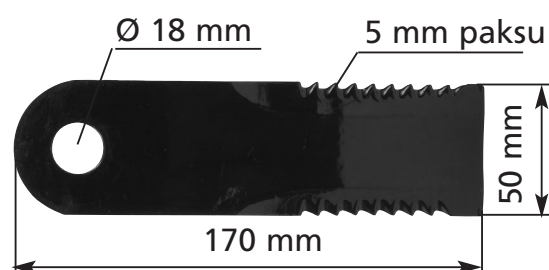
3605-0670-(OR) Pyörivä ja hammastettu terä Sopii KPAB:n silppurille
