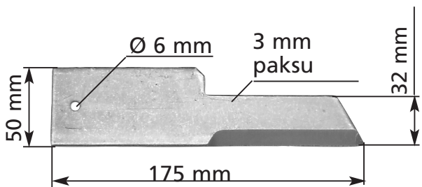
3605-0567 Vastaterä
