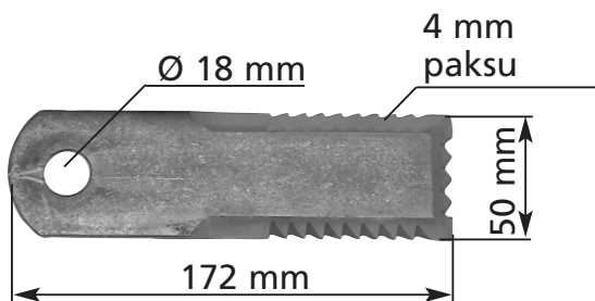
3605-0566-ORT Pyörivä terä, sivut ja pää hammastettu
