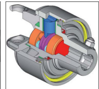
Nockenschaltkupplung lebensdauergerichtet doppelte Lagerung
