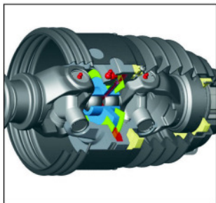
patentiertes 80° Weitwinkelgelenk
