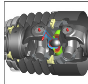
patentiertes 50° Weitwinkelgelenk
