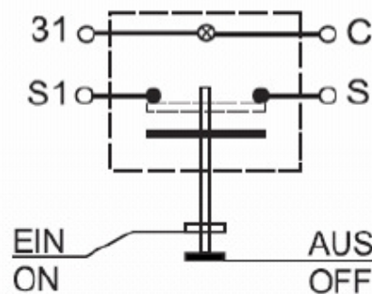
Schaltbild
