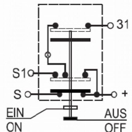
Schaltbild
