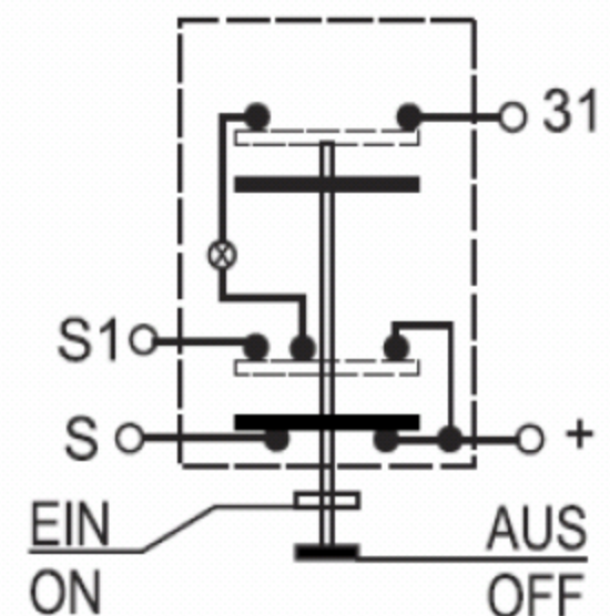
Schaltbild
