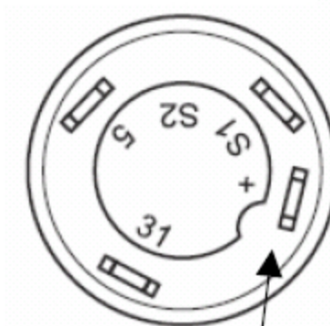
Steckeranordnung
