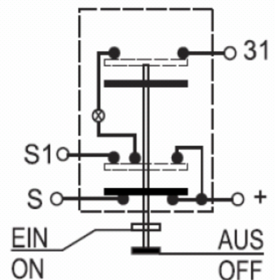
Schaltbild
