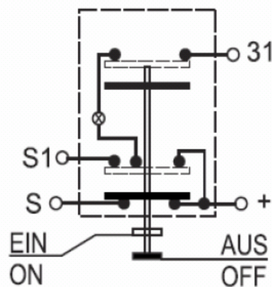
Schaltbild
