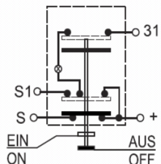
Schaltbild
