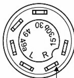
Stecker 6,3x0,8
