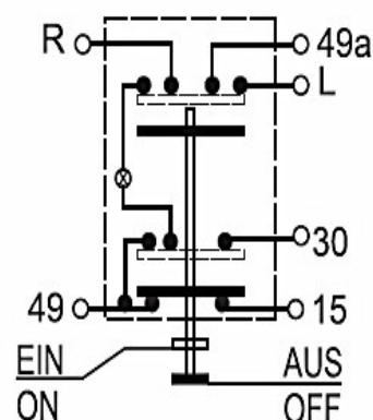
Schaltbild
