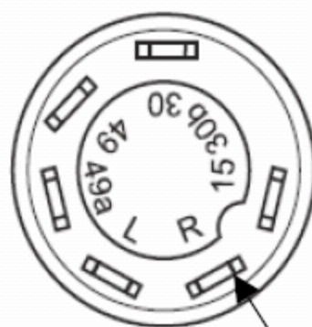
Steckeranordnung
