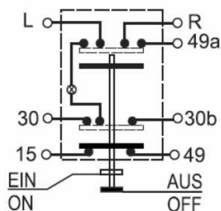
Schaltbild
