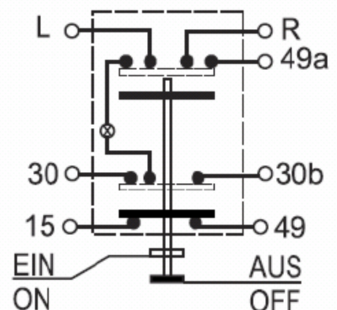
Schaltbild
