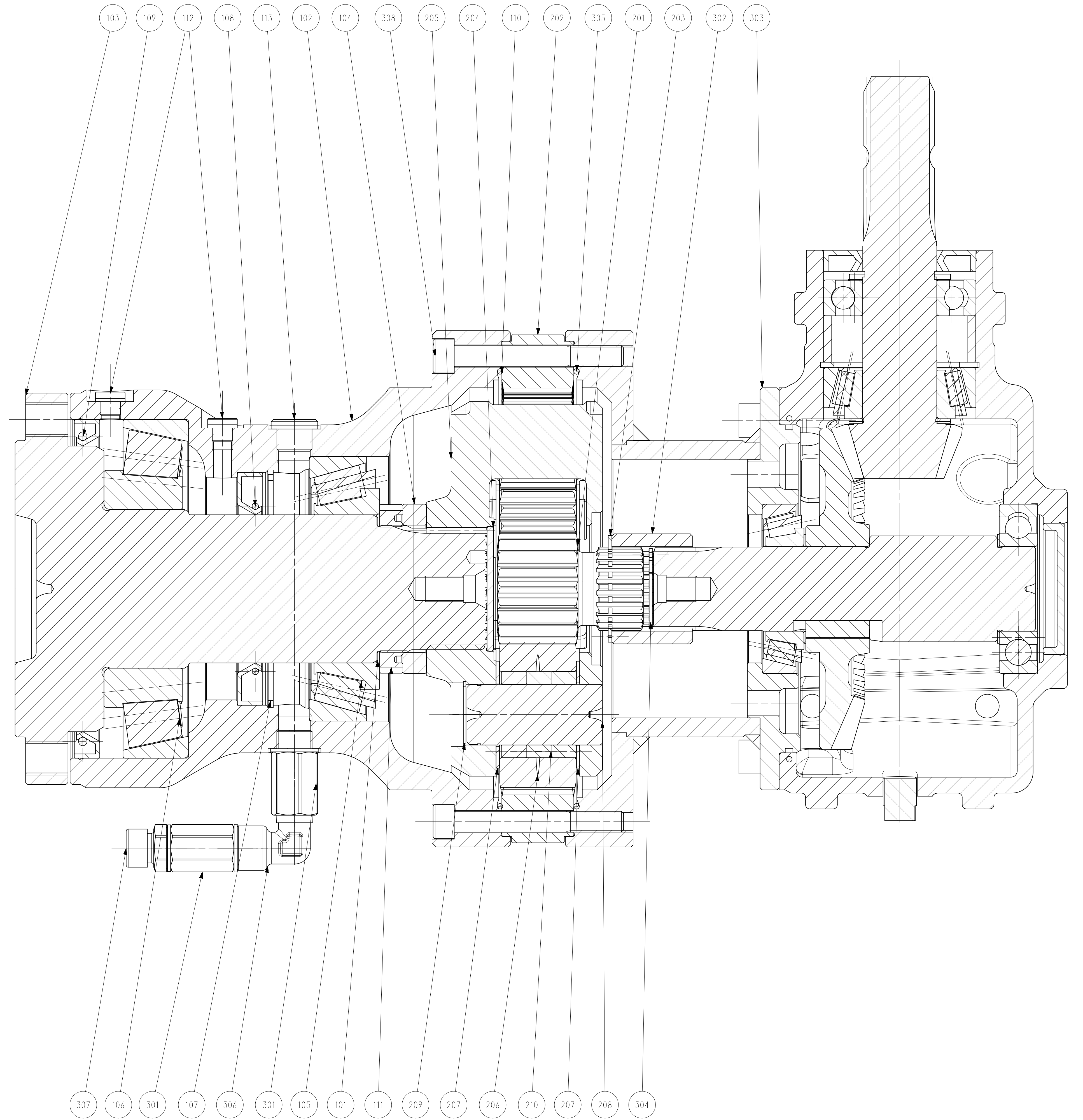
SEZ. / SECT. A-A
