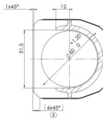
SNITT-DARSTELLUNG B-B
