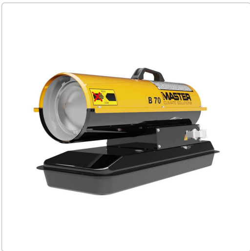
Master B 70 CED – direkte oliefyrede varmeapparater
