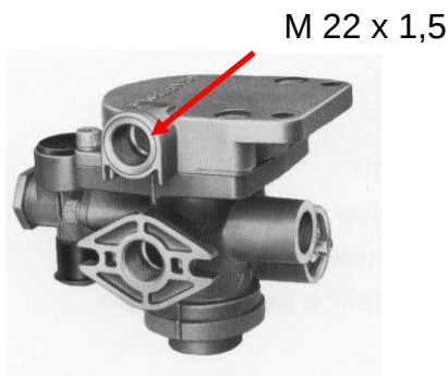
Anhängerbremssventil 1. Generation
