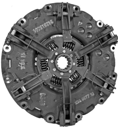
5 Paddle 228 0077 12 OEM 516 2897
