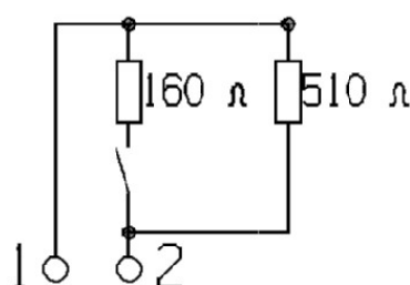
Schaltbild
