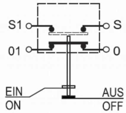
Schaltbild
