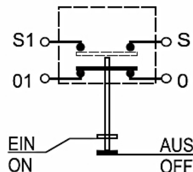
Schaltbild
