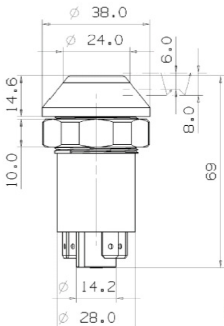
Steckeranordnung
