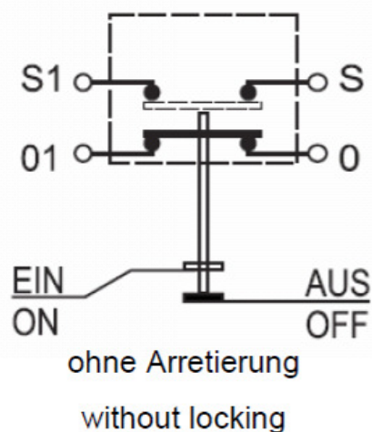
Schaltbild
