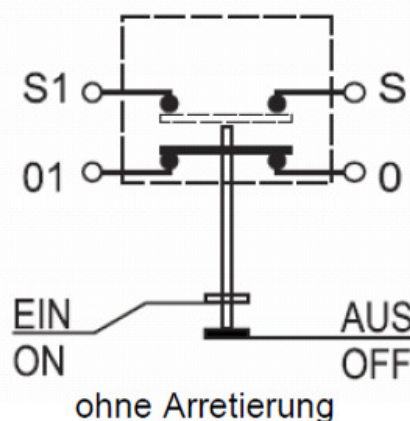
Schaltbild
