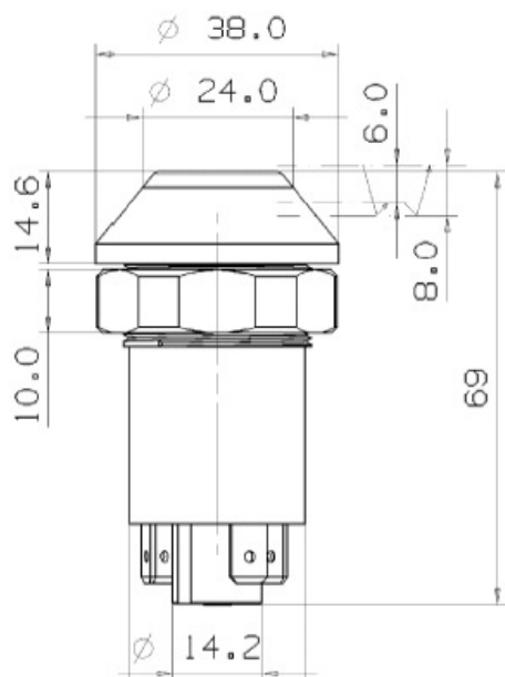
Steckeranordnung
