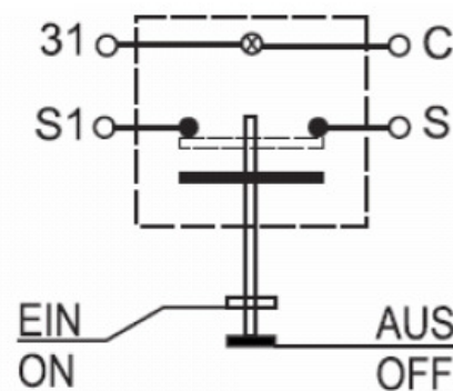
Schaltbild
