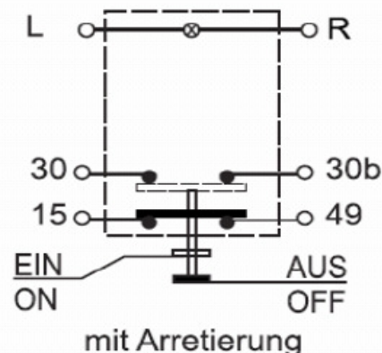
Schaltbild
