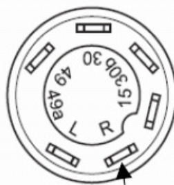
Steckeranordnung
