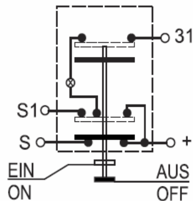
Schaltbild
