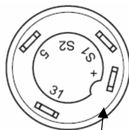
Steckeranordnung
