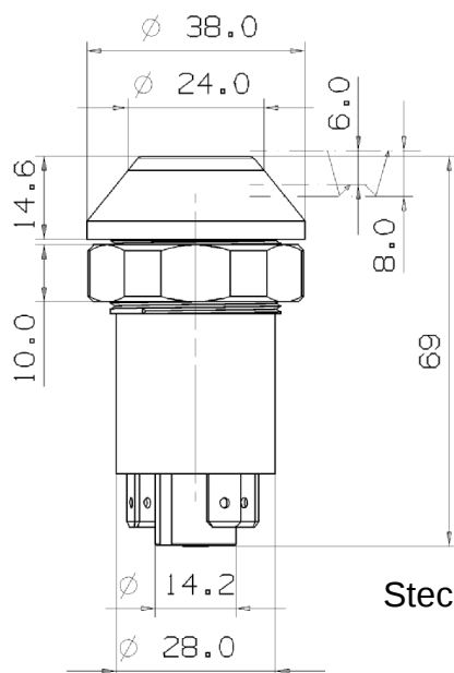
Steckeranordnung
