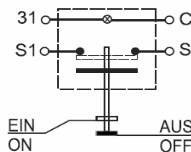
Schaltbild
